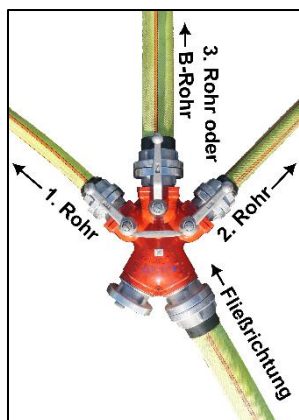
5.1-2 BB-CBC-Verteiler mit Kugelabsperrorganen
