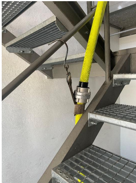
4.4.1-2 Entlastung der Schlauchleitung mittels eines Gurtschlauchhalters
