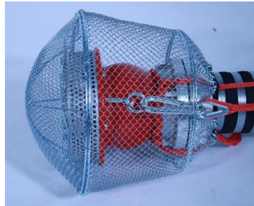
6.1-9 Saugschutzkorb am Saugkorb
