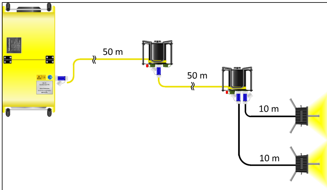
9.3.1-1 Schema Leitungslängen 100 Meter hintereinander
