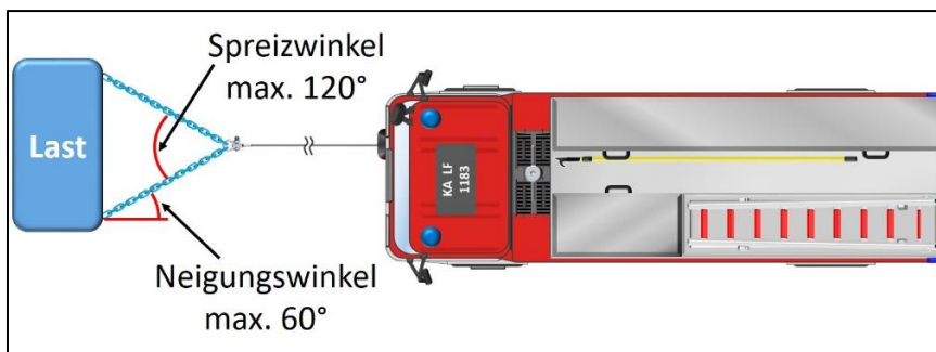
13.1-1 Spreiz- und Neigungswinkel
