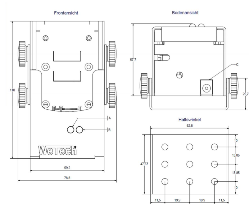
Schemazeichnung WTC680
